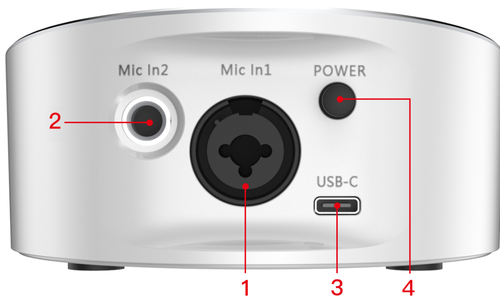
背面板接口
